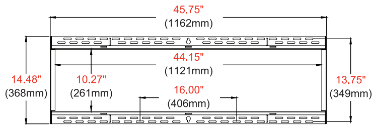
WANDPLATTEN-DETAILS
