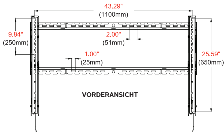
WANDPLATTEN-DETAILS
